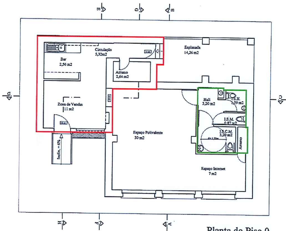
Planta do Piso 0
